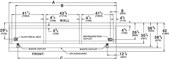
D5X-ULEP, D6X-ULEP Plan View
